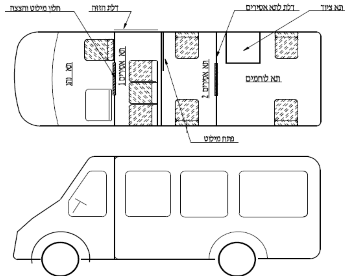
ציור מס.1: רכב להסעת 8 נוסעים + נהג
