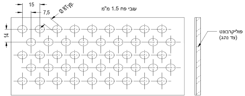
ציור מס. 2 : מחיצות: רשת + פוליקרבונט 3.5 מ"מ
