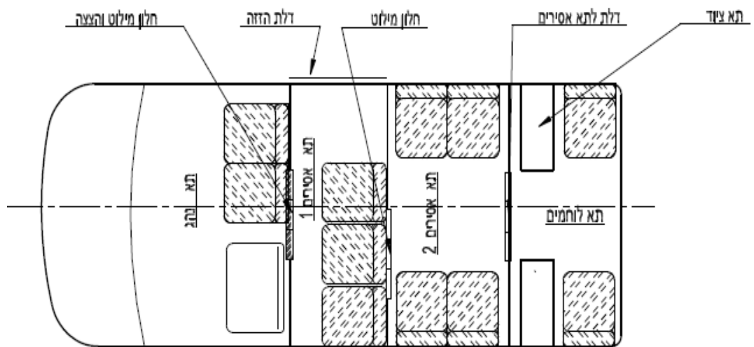
ציור מס.1 : מערך תאים
