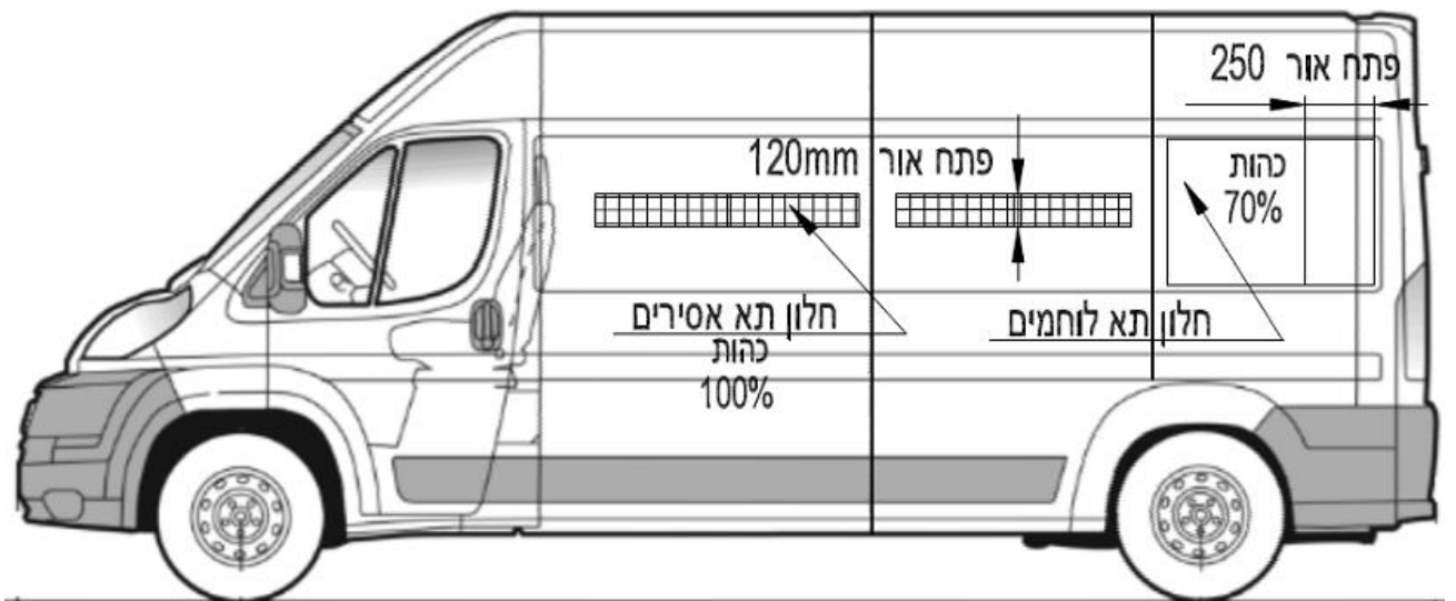
ציור מס. 3 : מערך חלונות
