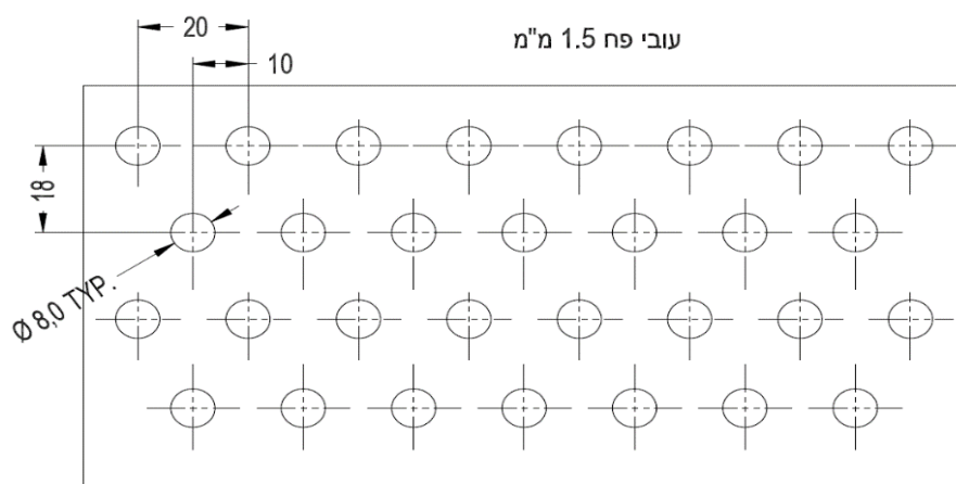
ציור מס.2 : רשת למזגן, תאורה וחלונות אסירים
